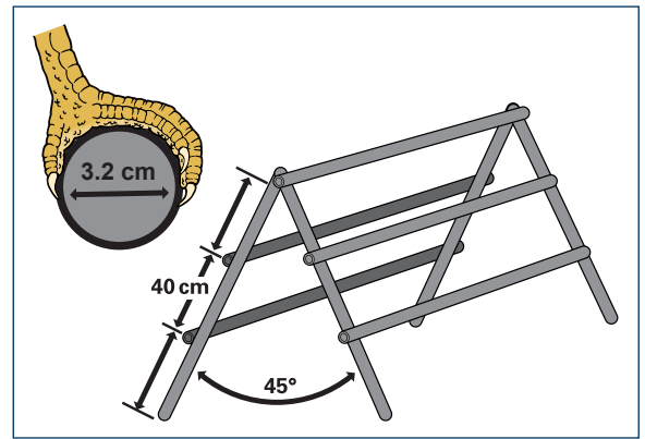
Насест А-формы
